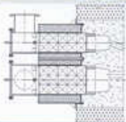
低热值双蓄热燃烧器 结构示意图
