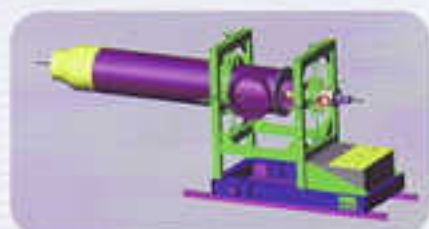
回转窑烧嘴及小车
