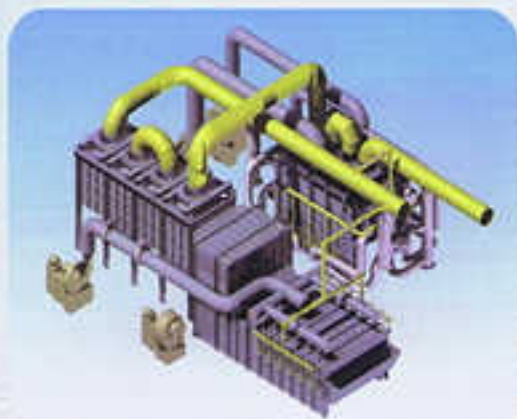
二级煤气预热炉 - 预热到900度
