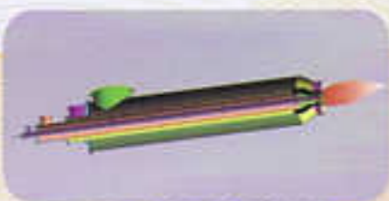
回转窑烧嘴半剖
