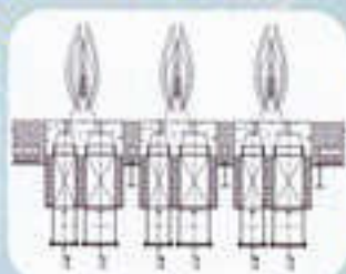
空煤气双预热水平交叉 流组合式蓄热式烧嘴
