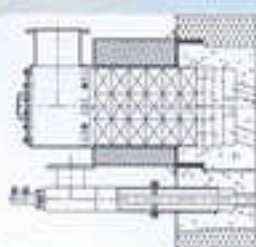
高热值单蓄热燃烧器结构示意图
